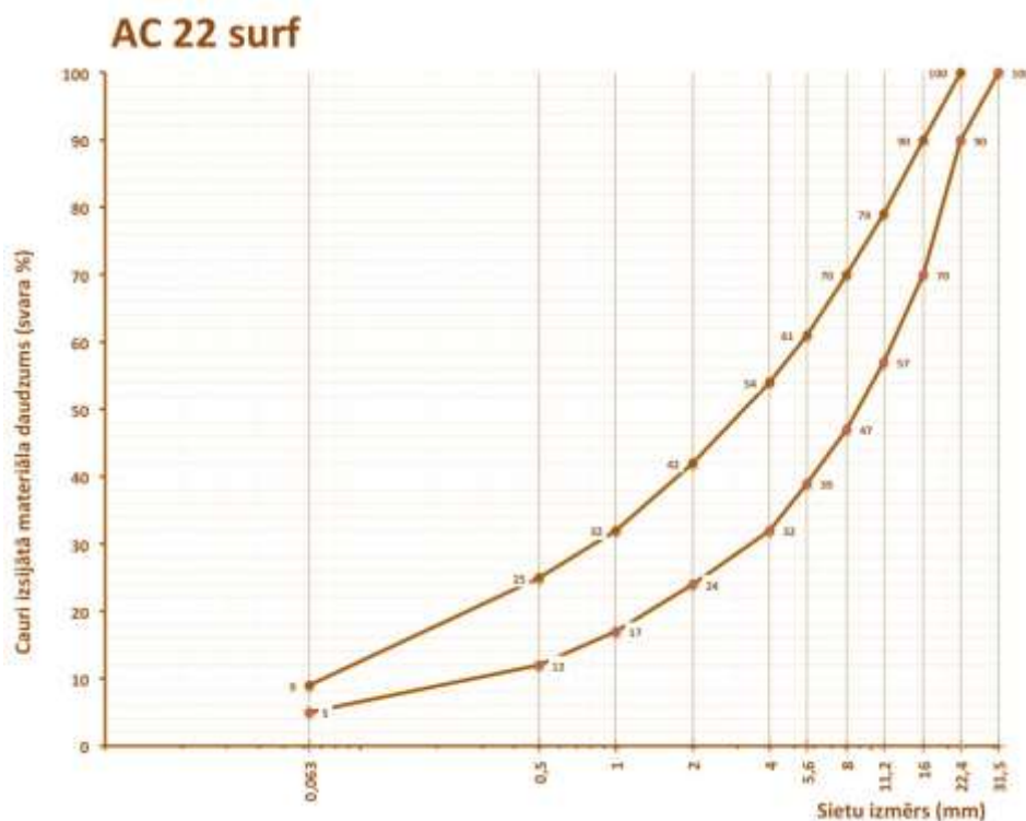
6.2-31 tabula. Prasības karstā asfalta AC 22 surf granulometriskajam sastāvam
